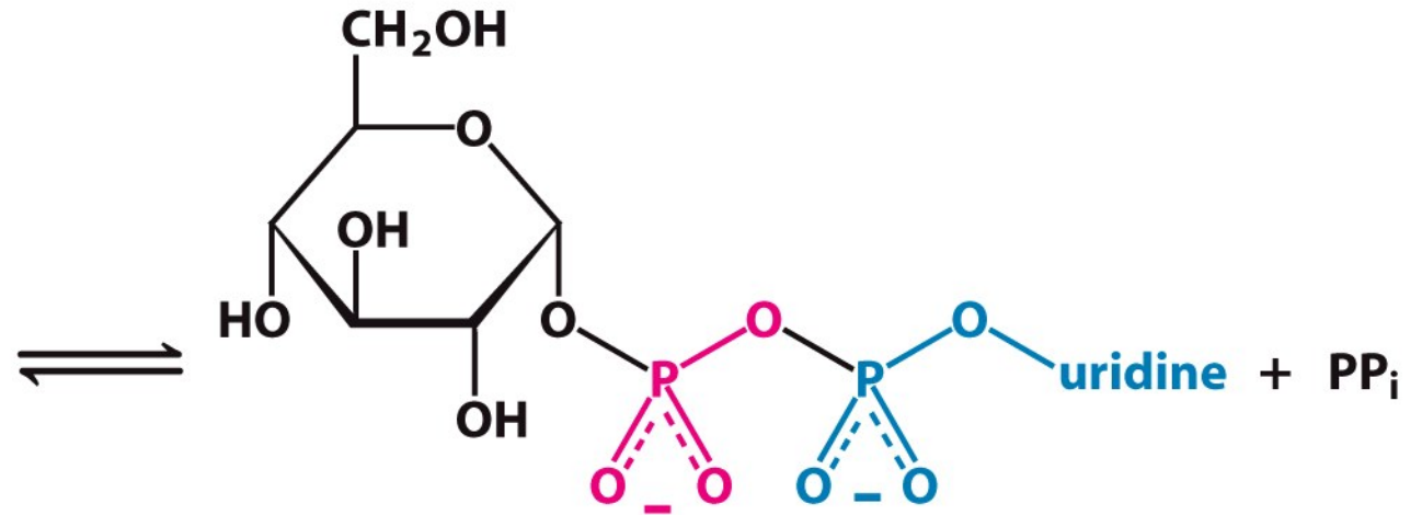
UDP-glucose
